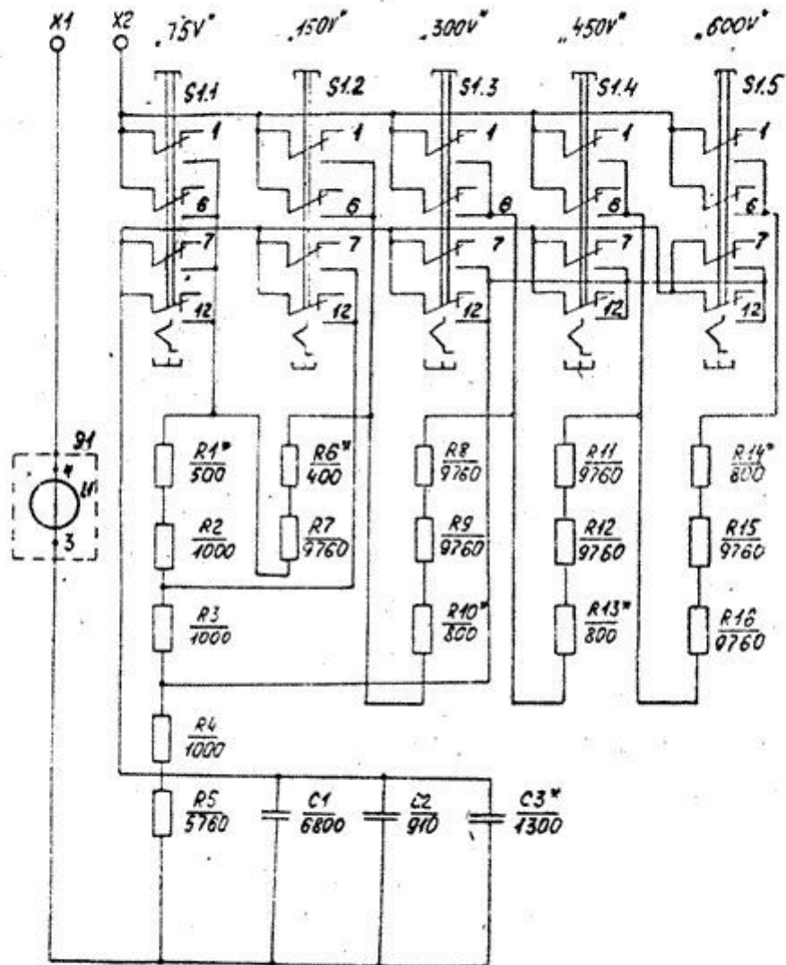
Вольтметр 3545, 3545-04.1. Схема электрическая принципиальная
